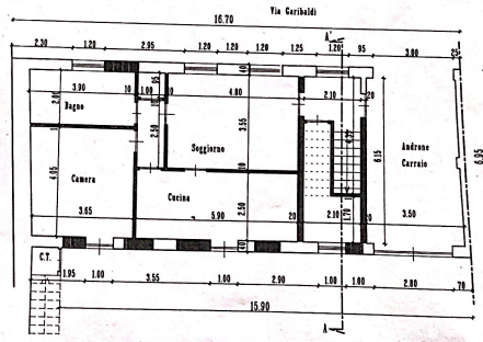
Pianta Piano Terra in Progetto
