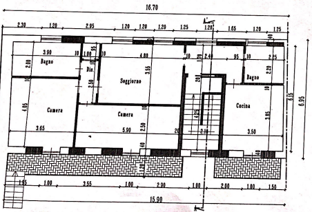
Pianta Piano Primo in Progetto
