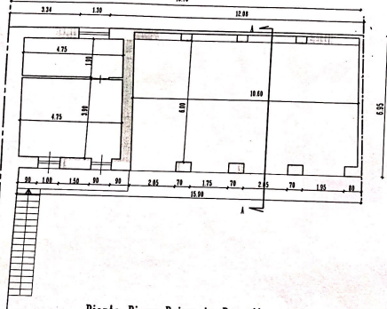
Pianta Piano Primo in Progetto
