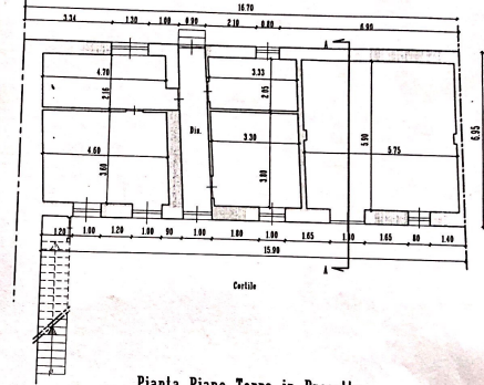
Pianta Piano Terra in Progetto
