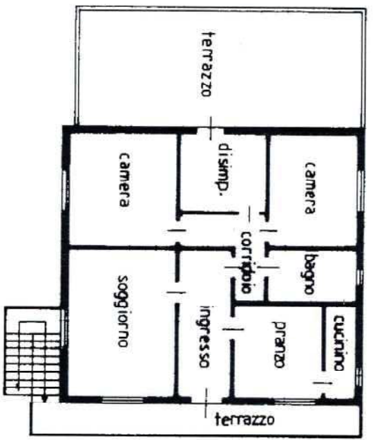
PIANTA PIANO PRIMO H = 2.85
