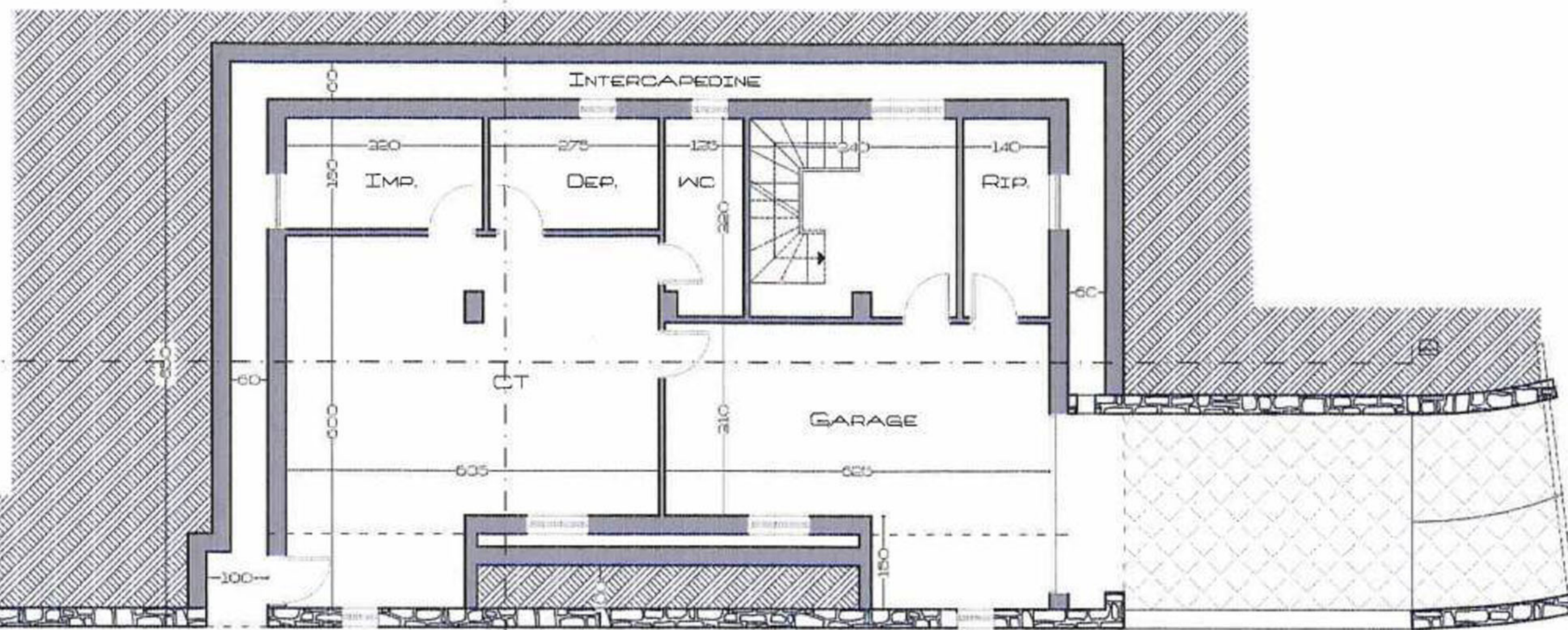
PIANTA PIANO INTERRATO
