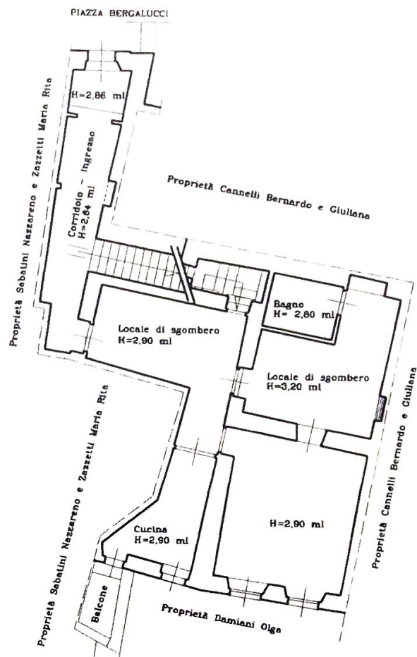
PIANTA PIANO TERRA 76,77 mq netti senza scala 113,68 mq lordo 2,28 mq balcone netto 3,79 mq balcone lordo
