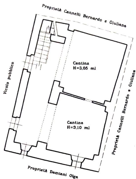
PIANTA PIANO SEMINTERRATO 54,67 mq netti senza scala 80,80 mq lordo
