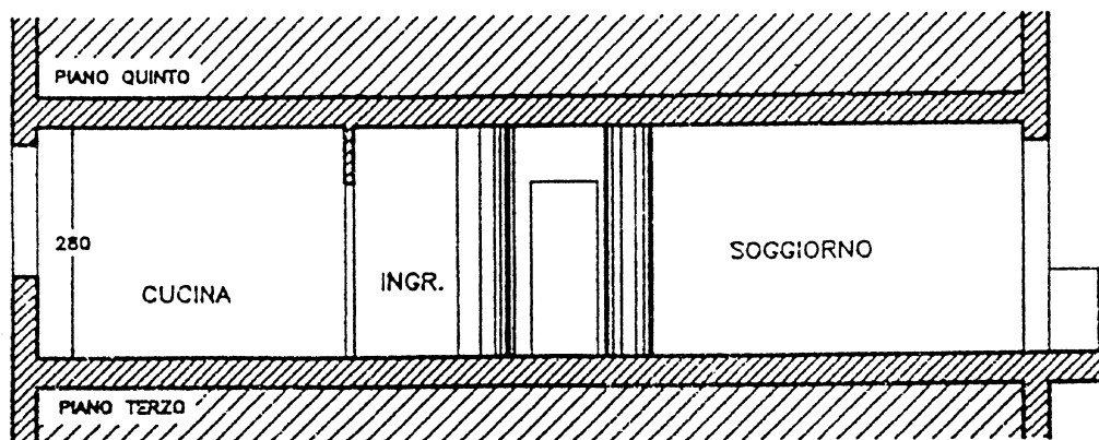
SEZIONE A-A
