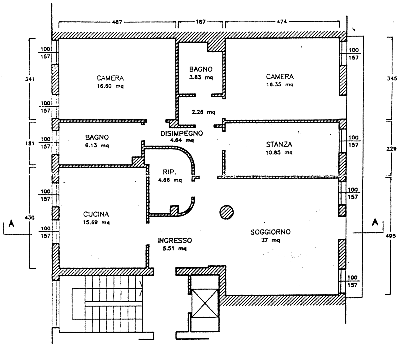
PIANTA PIANO QUARTO H 280
