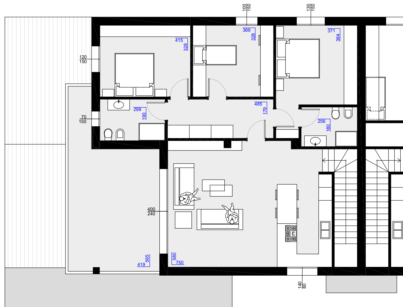
PIANO PRIMO
