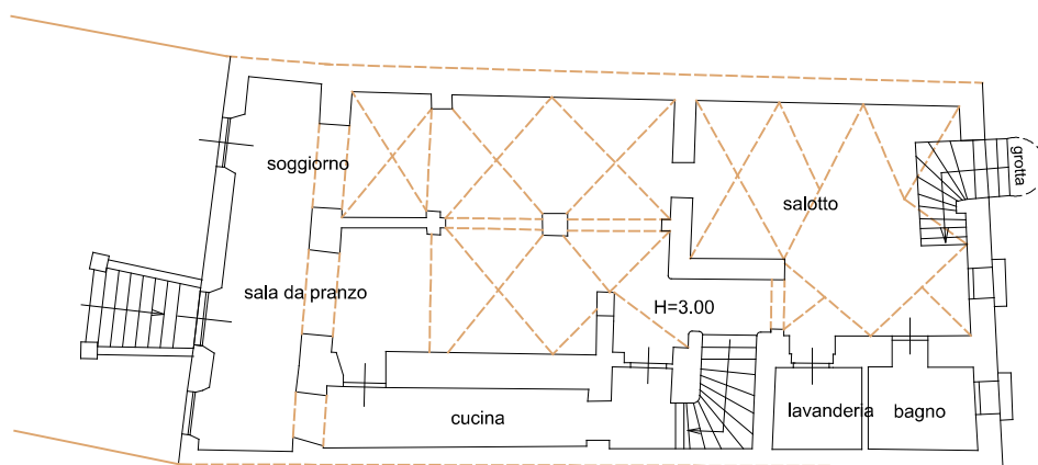
Piano Terra - PT
