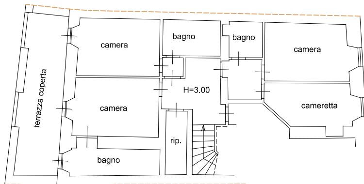
Piano Terra - PT
