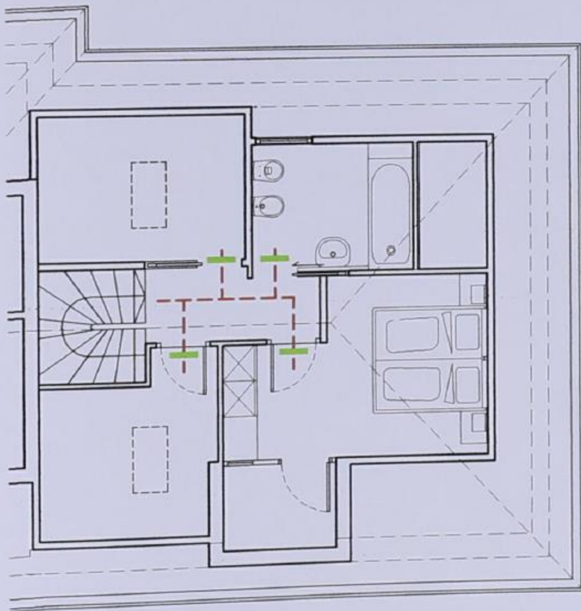
DACHGESCHOSS - 1:100
