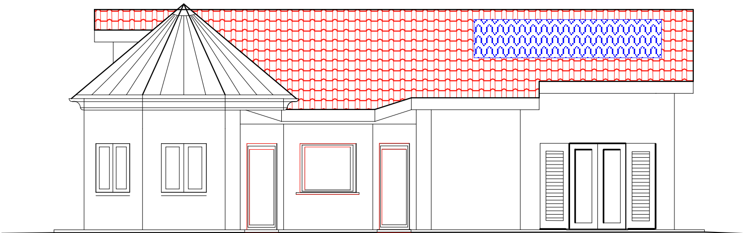
PROSPETTO SUD
