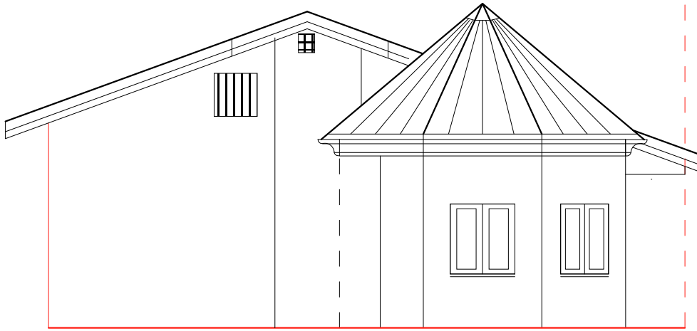
PROSPETTO OVEST
