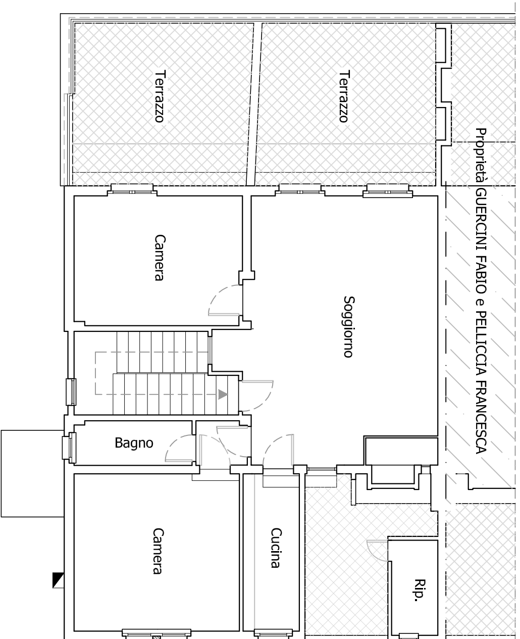
Pianta Piano SECONDO Scala 1:100
