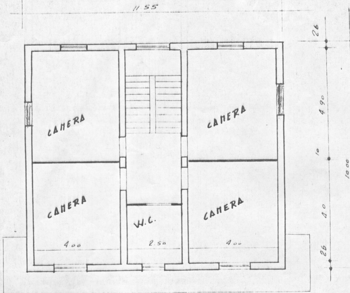
PIANO PRIMO
