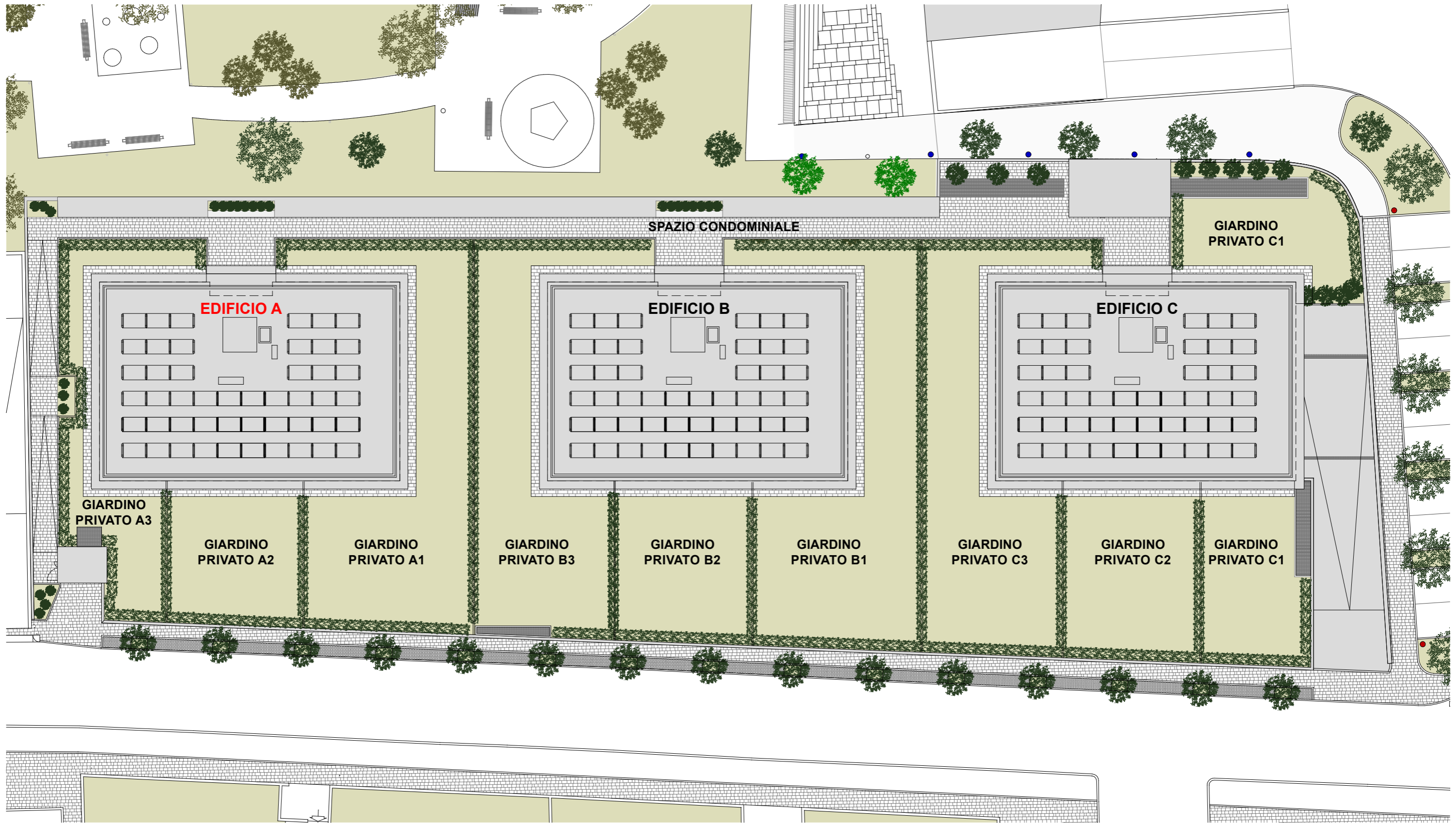
PLANIMETRIA GENERALE
