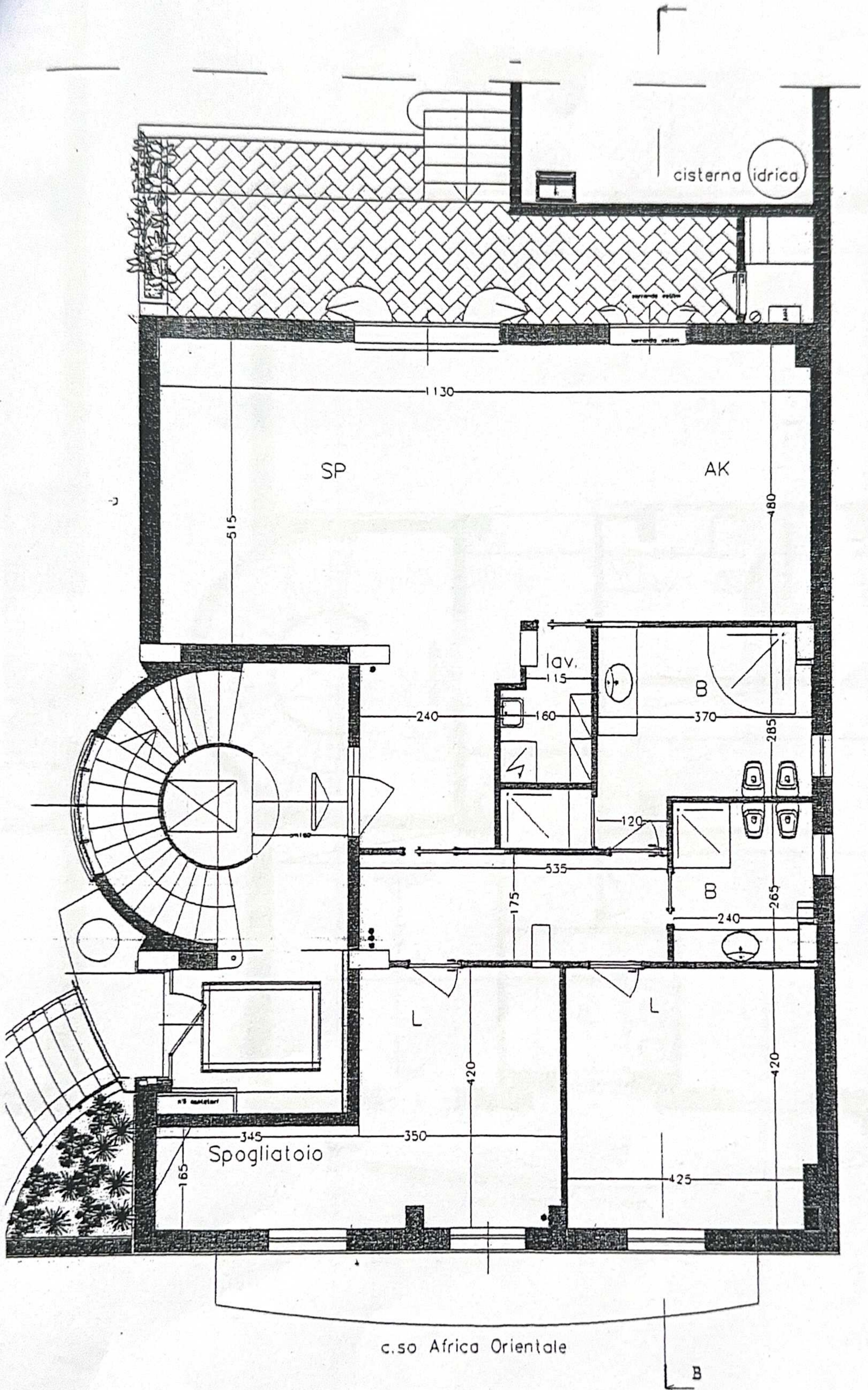
pianta piano rialzato
