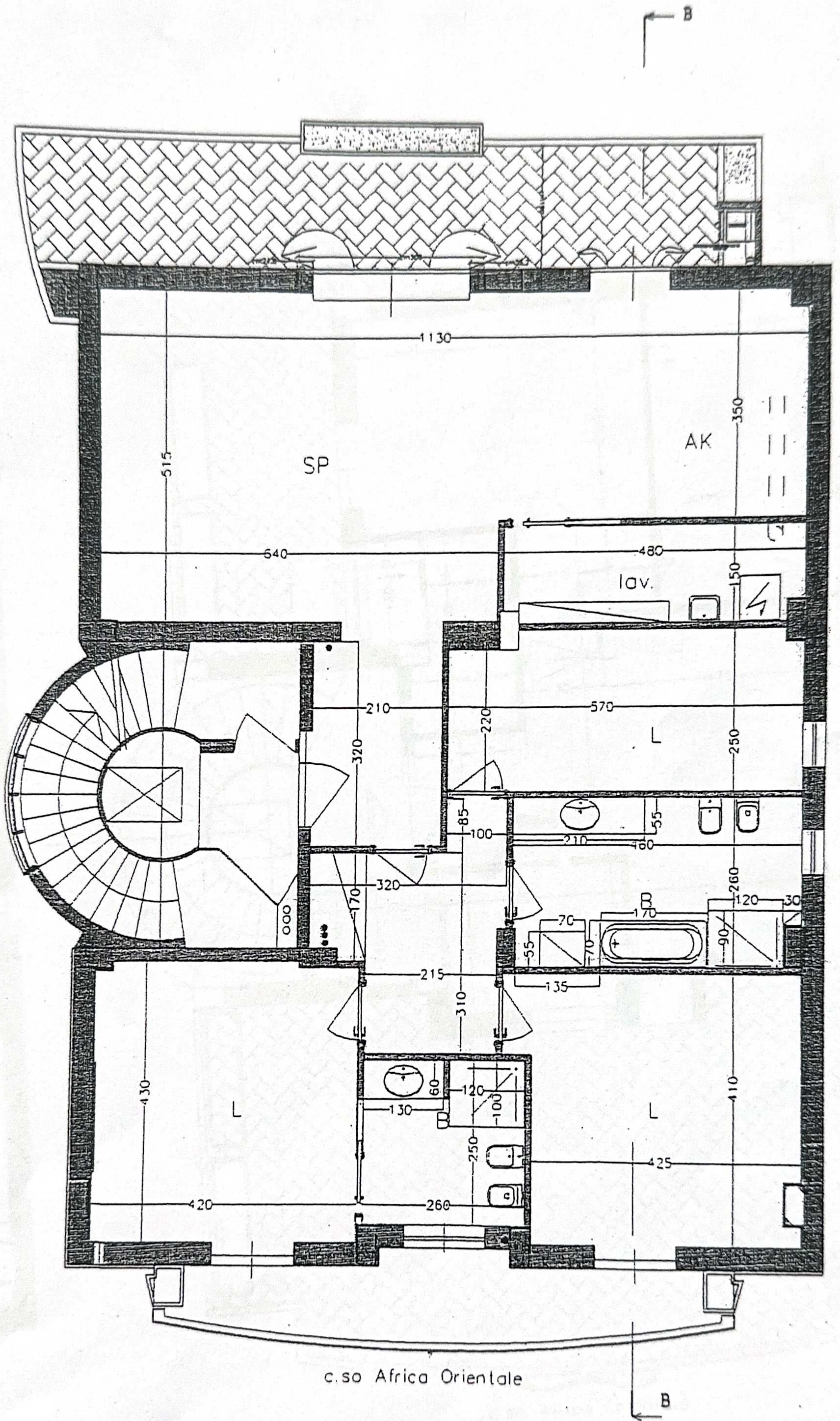
pianta piano secondo
