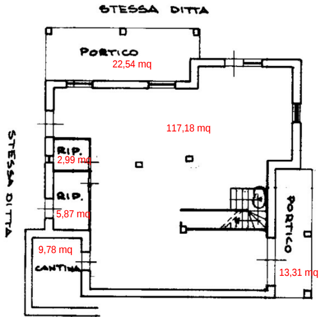
PIANO SOTTOSTRADA H= MT. 2.80
