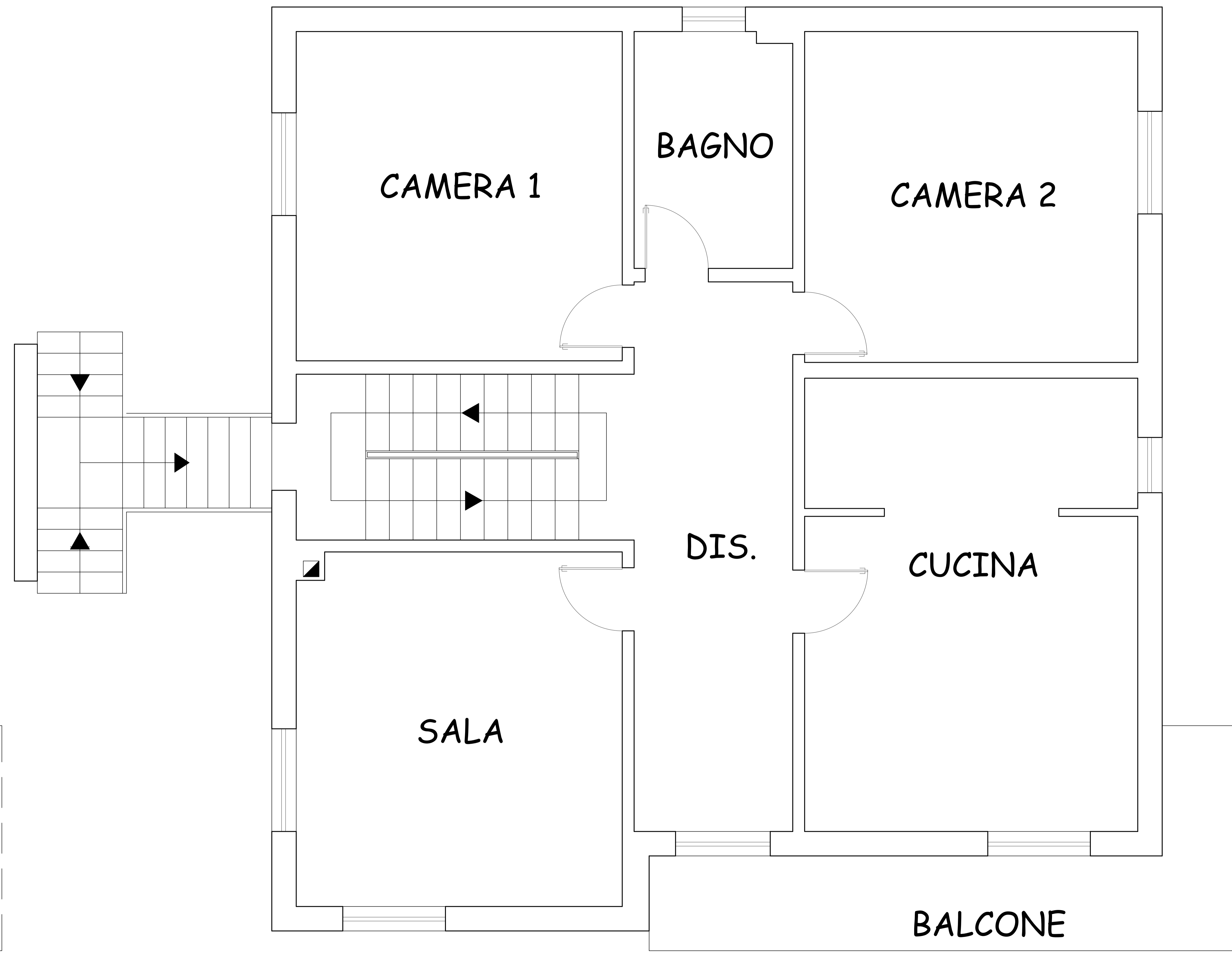
PIANO PRIMO
