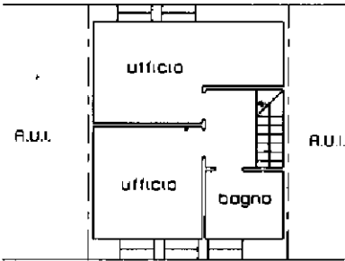
PIANO TERZO h medio 2.70
