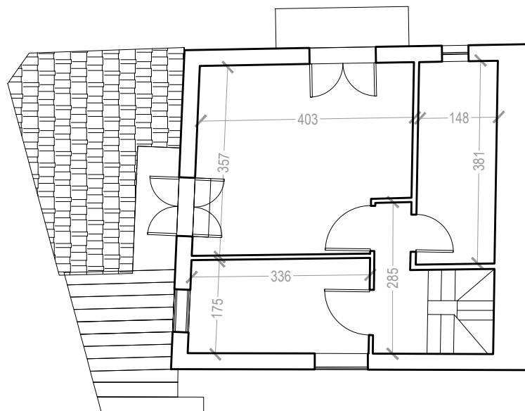
PIANTA 2° PIANO
