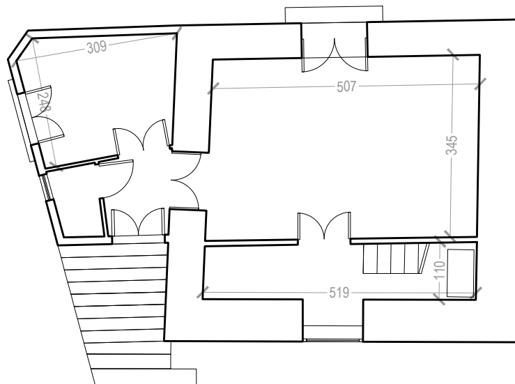
PIANTA 2° PIANO
