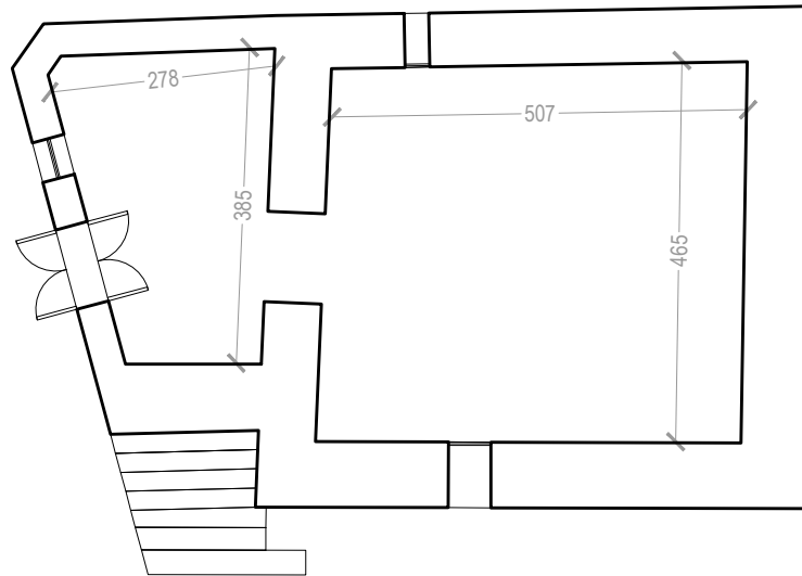
PIANTA 1° PIANO
