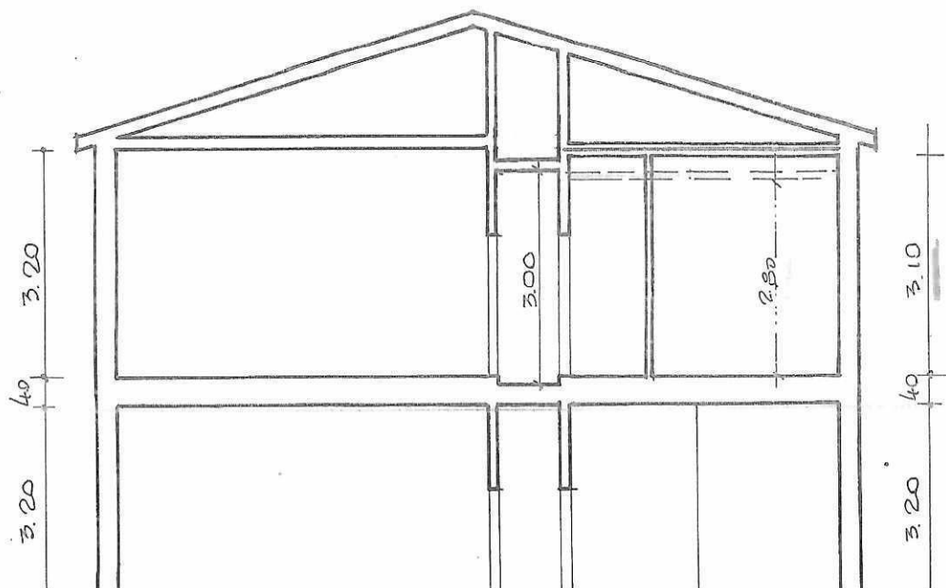
SEZIONE
