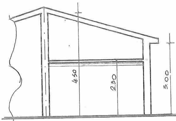
SEZIONE
