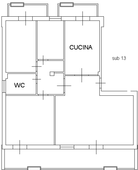
Piano Secondo H=2,93
