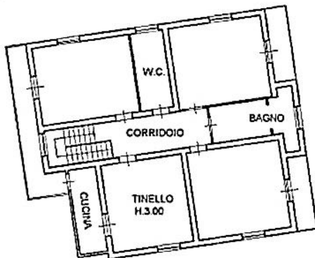
Piano Primo
