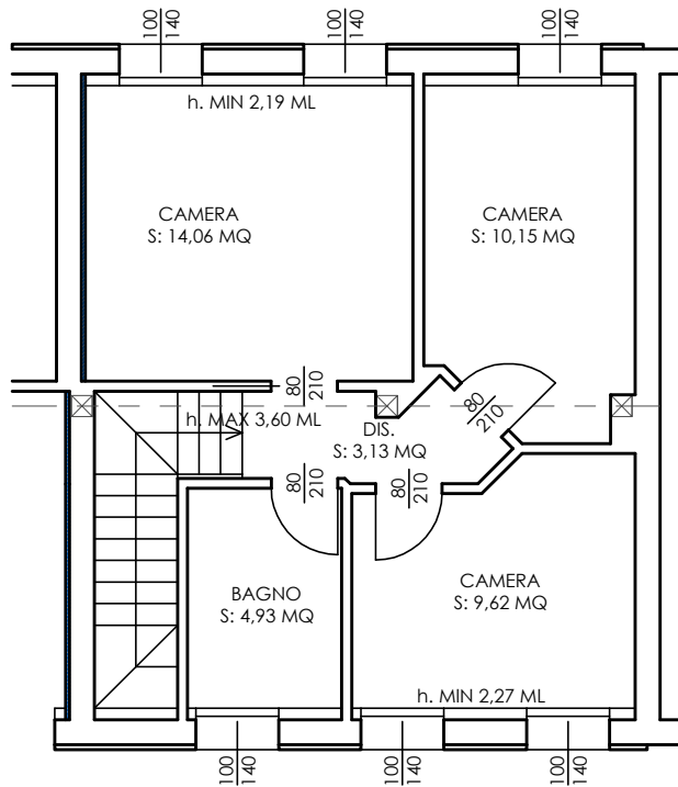
PIANO PRIMO Scala 1:100
