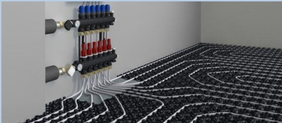
Esempio: impianto di raffrescamento a pavimento
