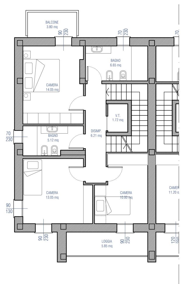
PIANO PRIMO
