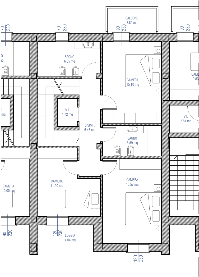
PIANO PRIMO
