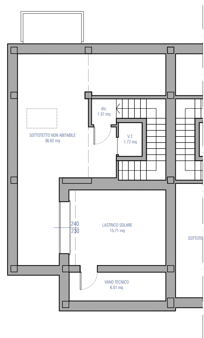
PIANO SOTTOTETTO
