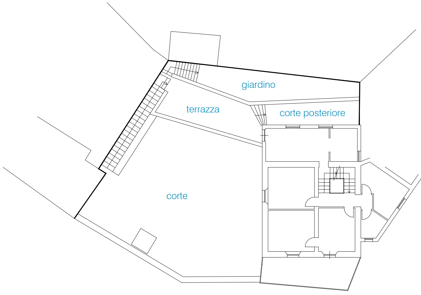
planimetria generale - scala 1:200 a livello mezzanino tra piano primo e secondo
