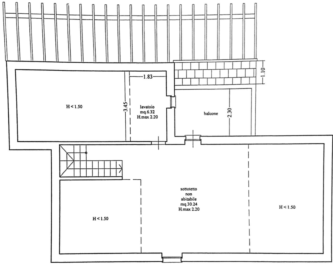
PIANO SOTTOTETTO
