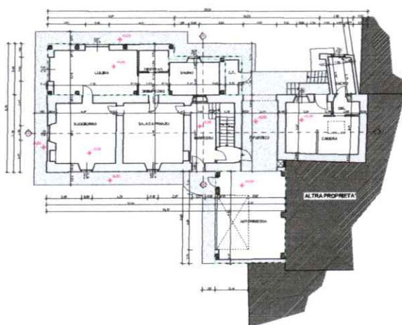
PIANTA PIANO PRIMO - progetto 1:100
