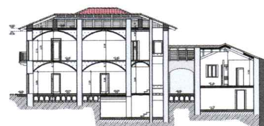
SEZIONE A/A - progetto 1:100
