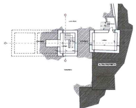
PIANTA PIANO INTERRATO - progetto 1:100
