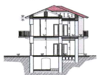
SEZIONE B/B - progetto 1:100
