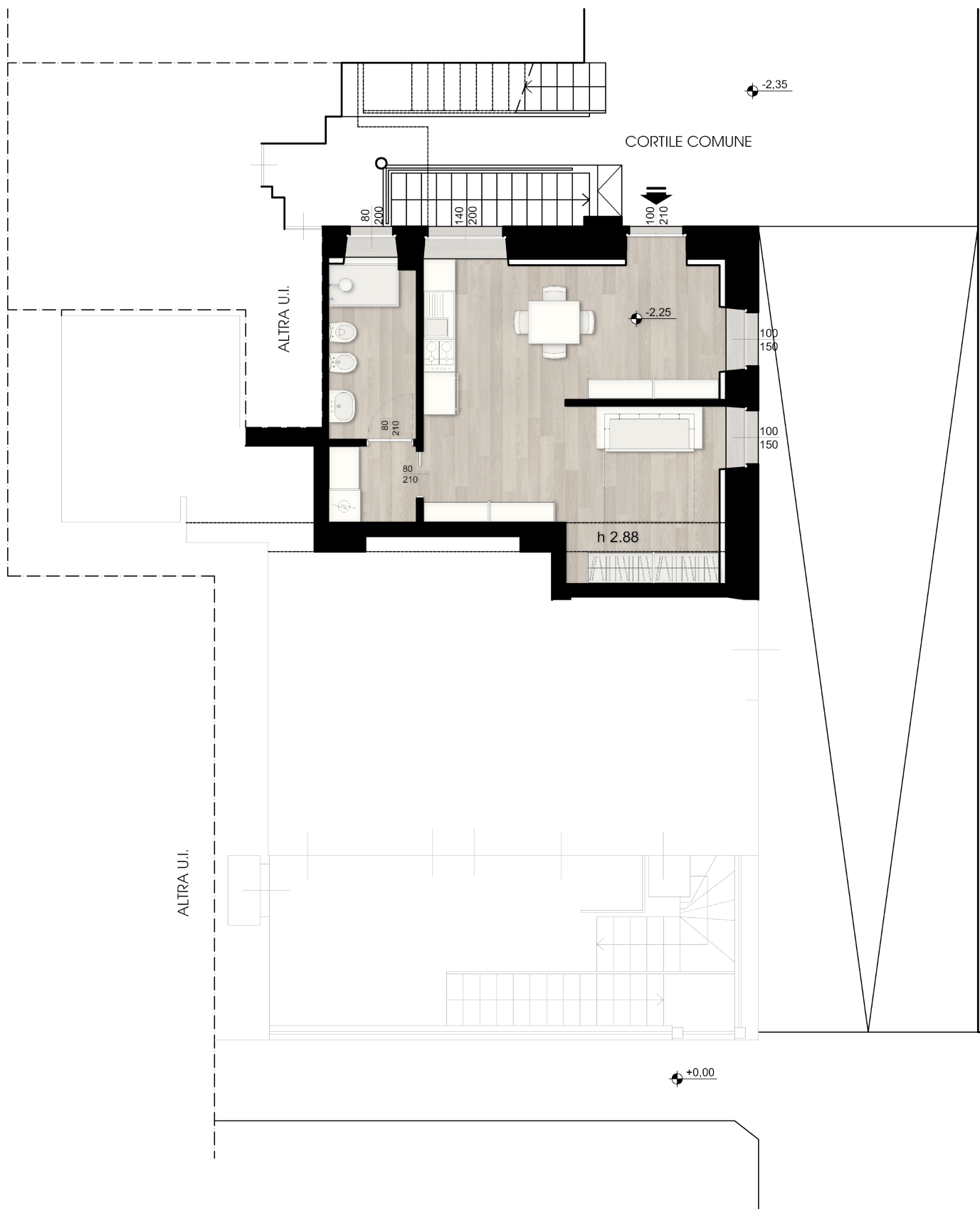
PIANTA PIANO SEMINTERRATO - PROPOSTA MONOLOCALE
