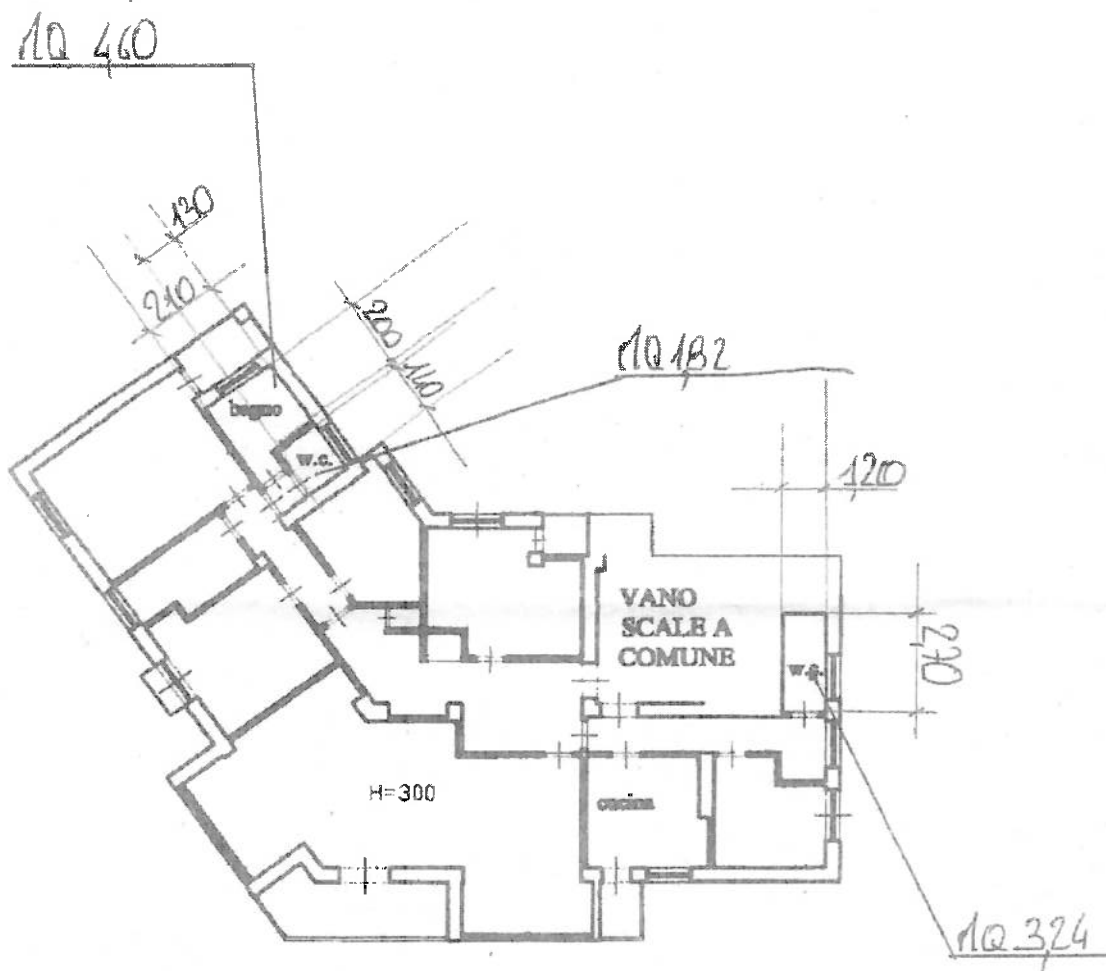
PIANTA PIANO SETTIMO
