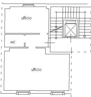
PIANO SECONDO h=3,35 mt.
