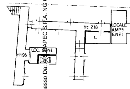
PIANTA PIANO INTERRATO
