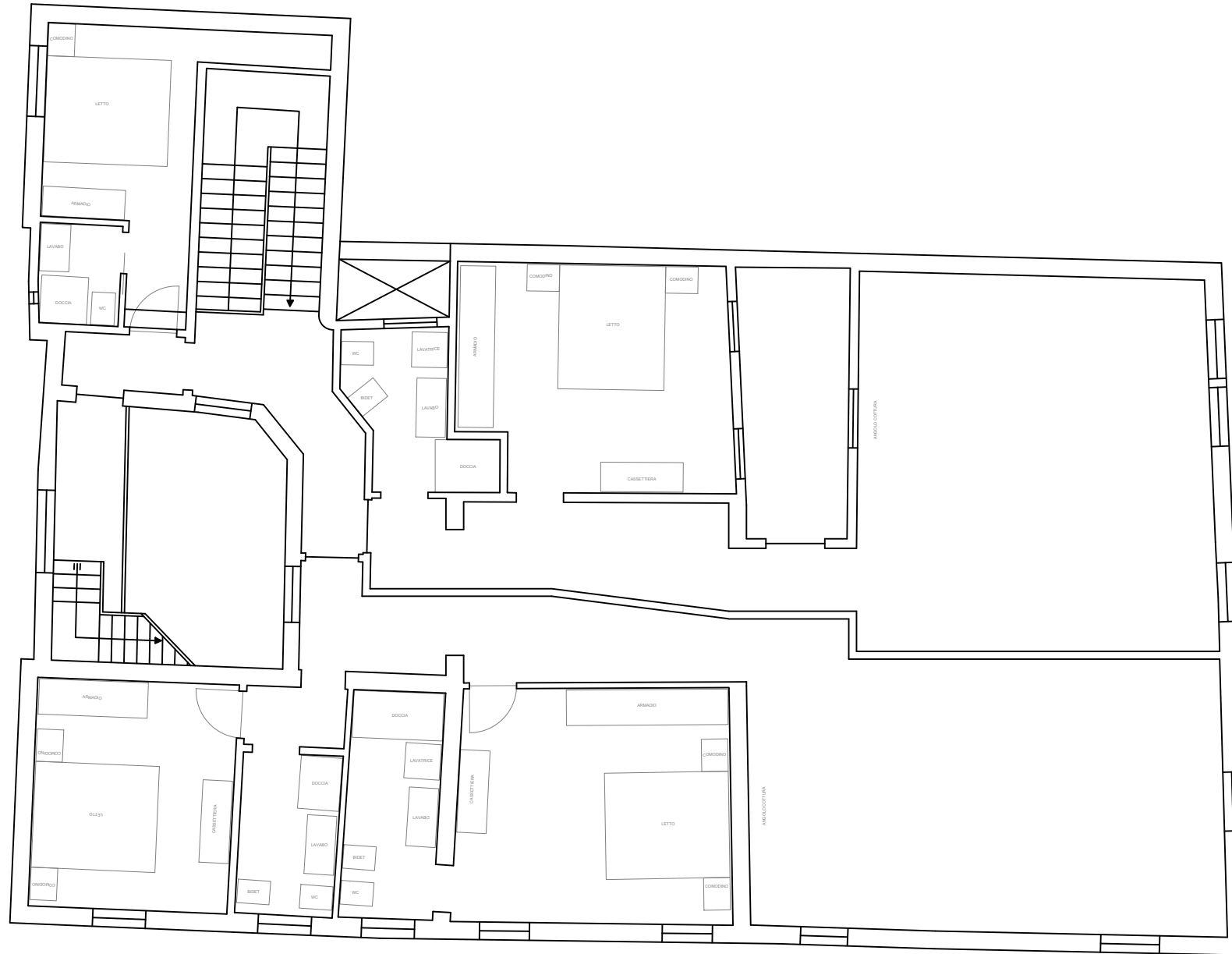
PIANO SECONDO
