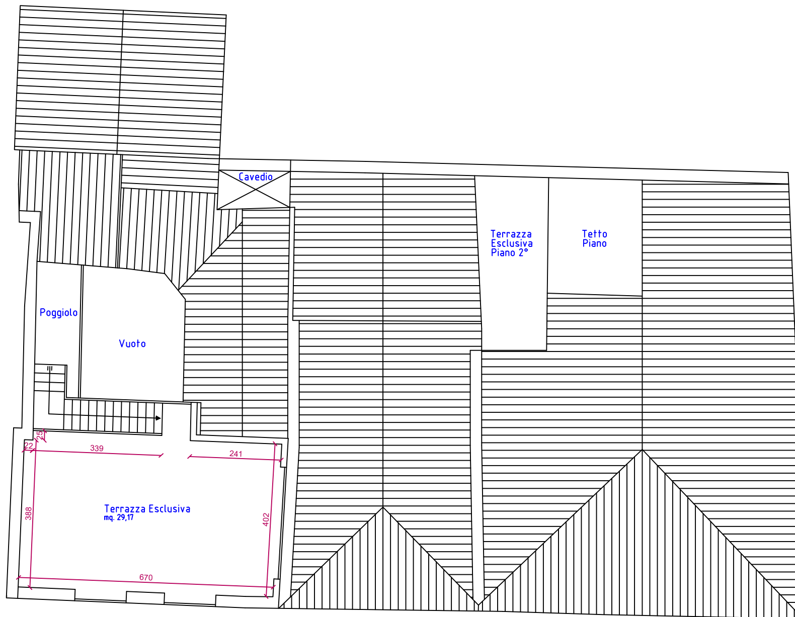
PIANO COPERTURA
