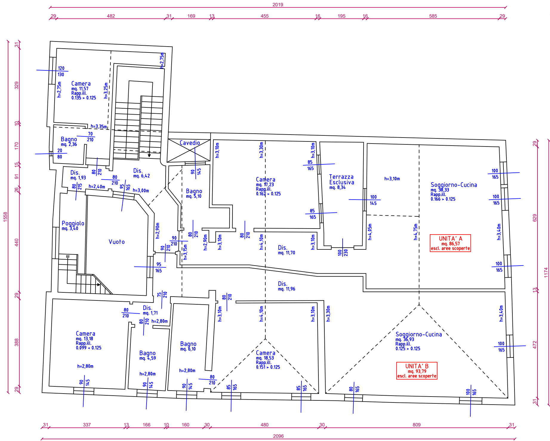
PIANO SECONDO
