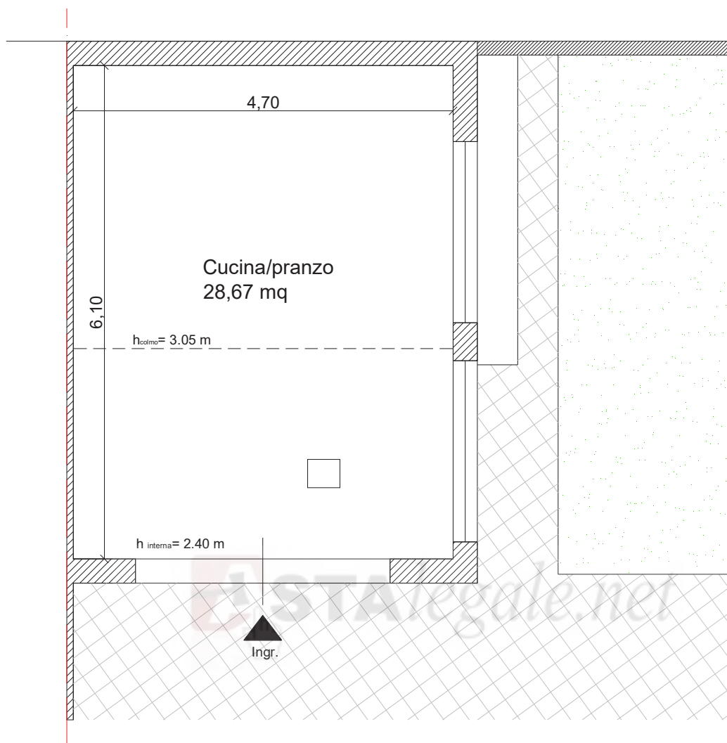
PLANIMETRIA DELL'UNITA' 1 -(fuori scala)
