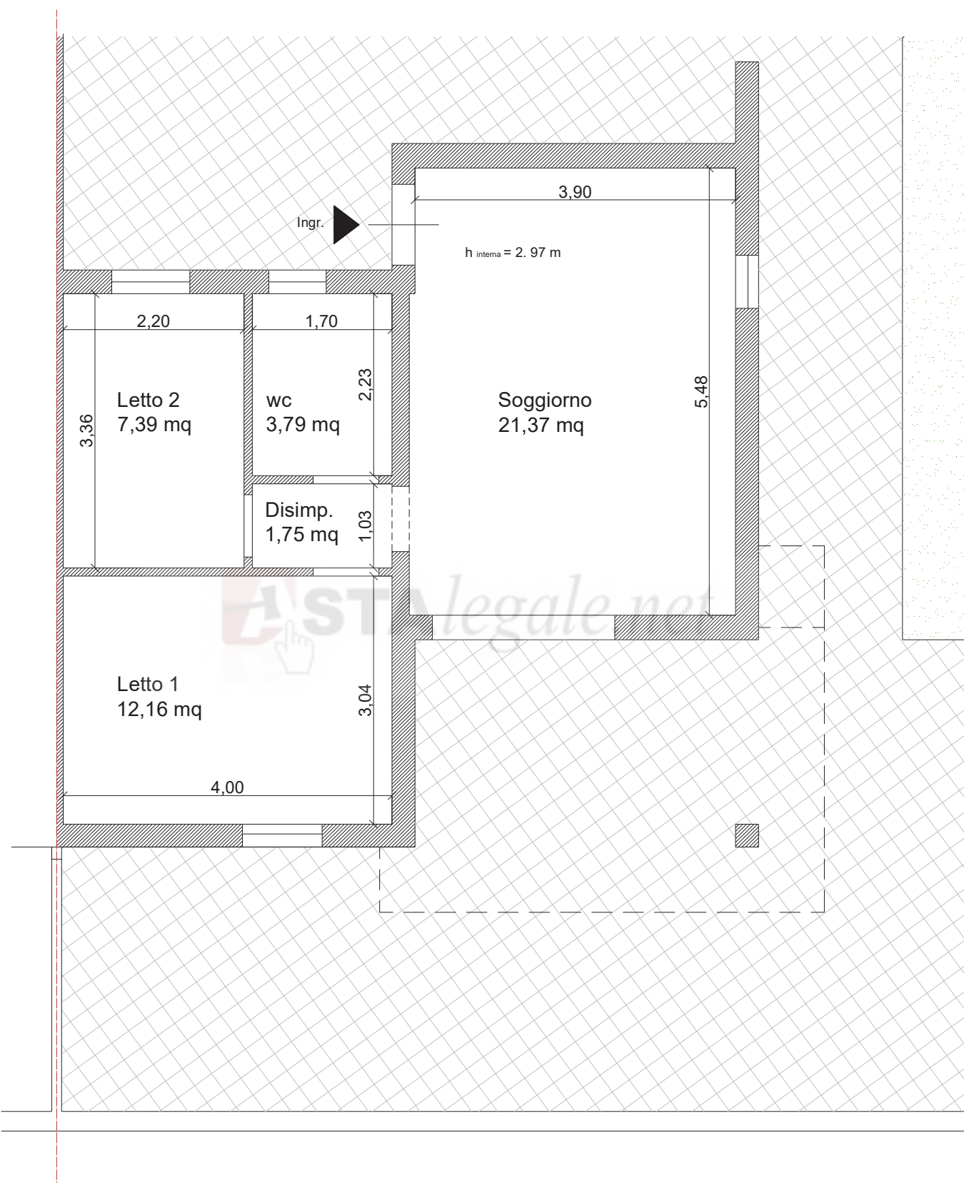
PLANIMETRIA DELL'UNITA' 2 - (fuori scala)
