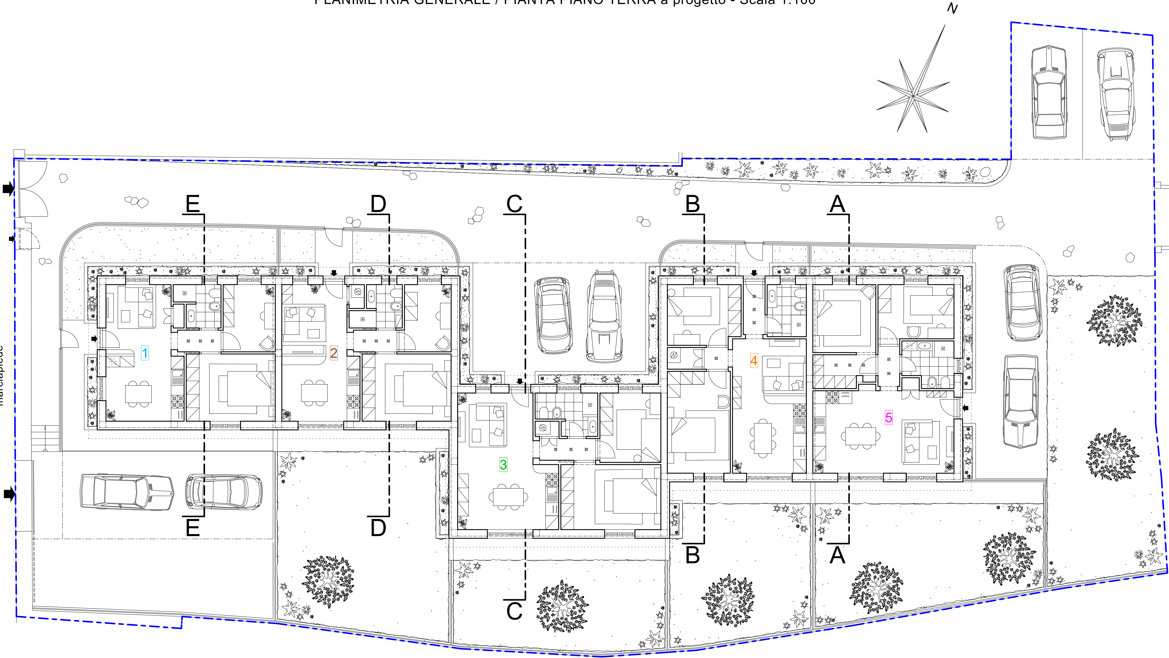
PLANIMETRIA GENERALE / PIANTA PIANO TERRA a progetto - Scala 1:100
