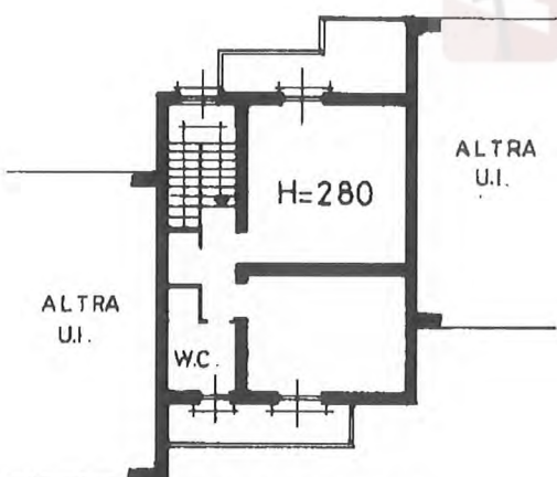
PIANO PRIMO
