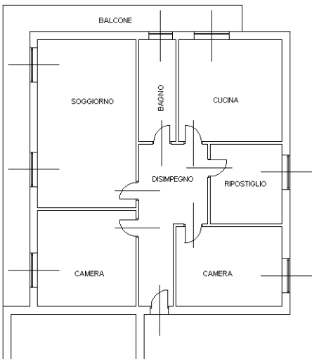
PIANTA PIANO PRIMO H=2,70
