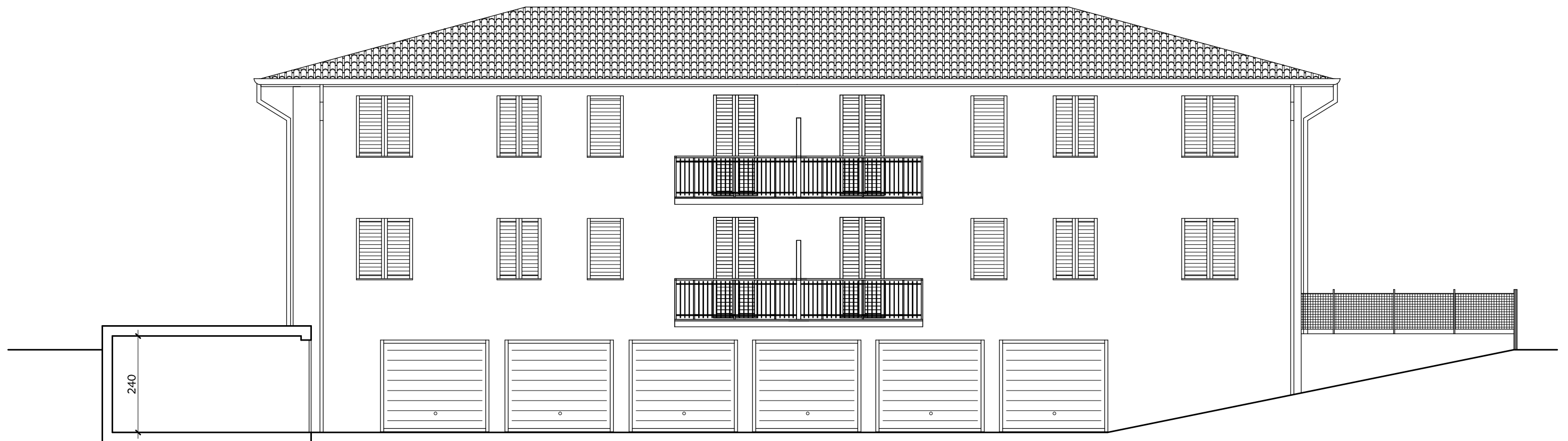
Prospetto Est
