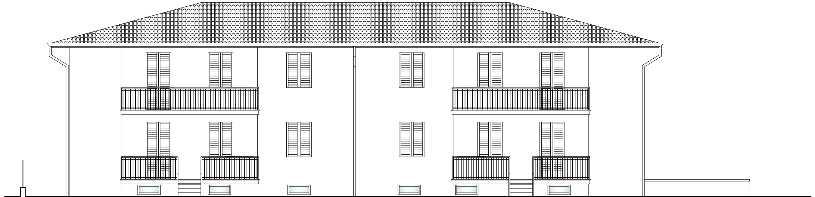
Prospetto Ovest
