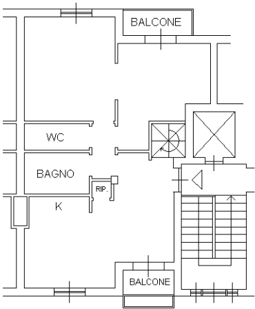
PIANO SECONDO ( H = 2,70 mt )
