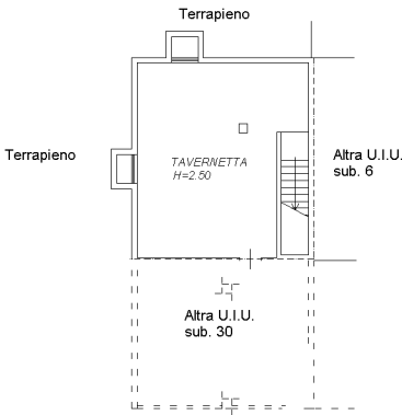
PIANTA PIANO PRIMO SOTTERRANEO
