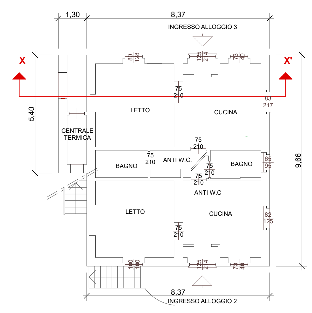
PLANIMETRIA ESISTENTE PIANO TERRENO scala 1/100
