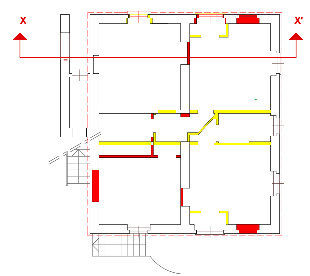
PLANIMETRIA COMPARATIVA PIANO TERRENO scala 1/100
