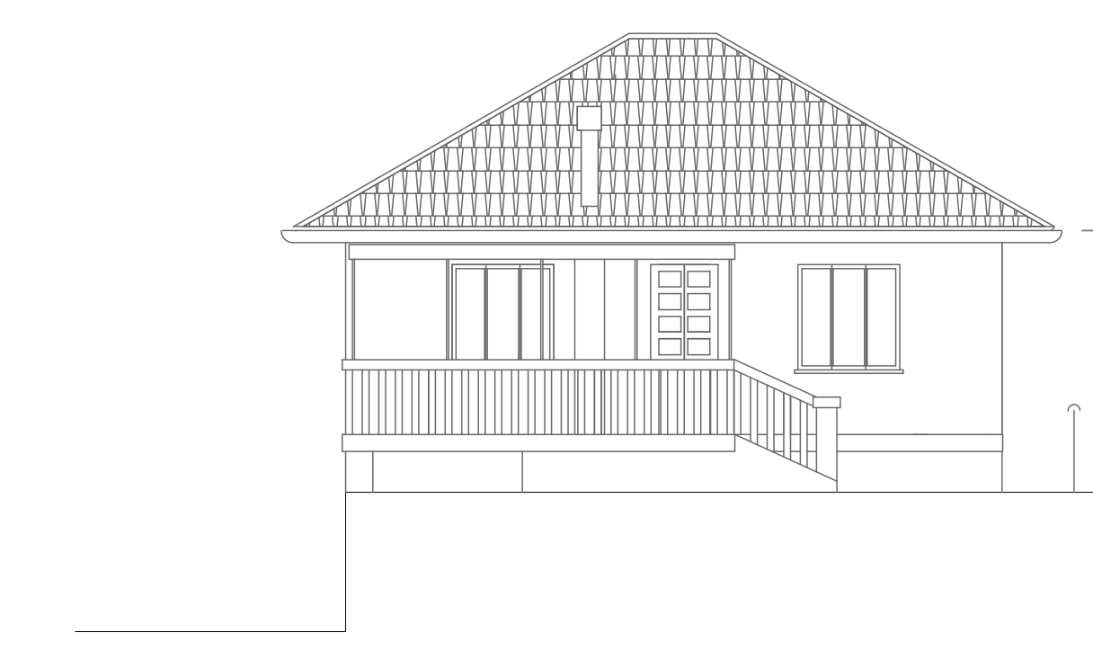
PROSPETTO OVEST ESISTENTE scala 1/100
