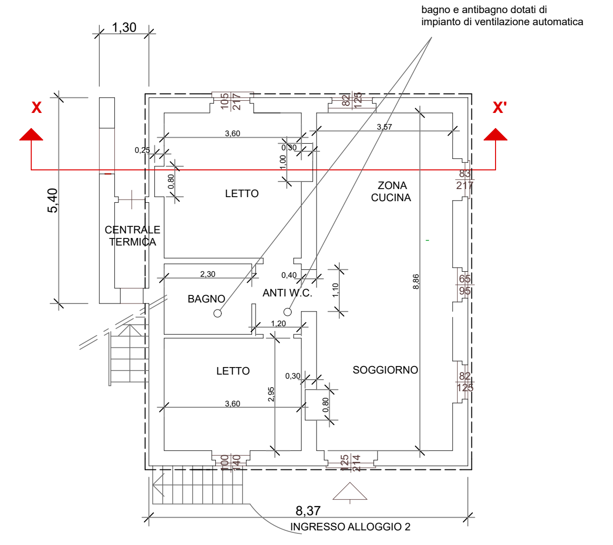
PLANIMETRIA IN PROGETTO PIANO TERRENO scala 1/100
