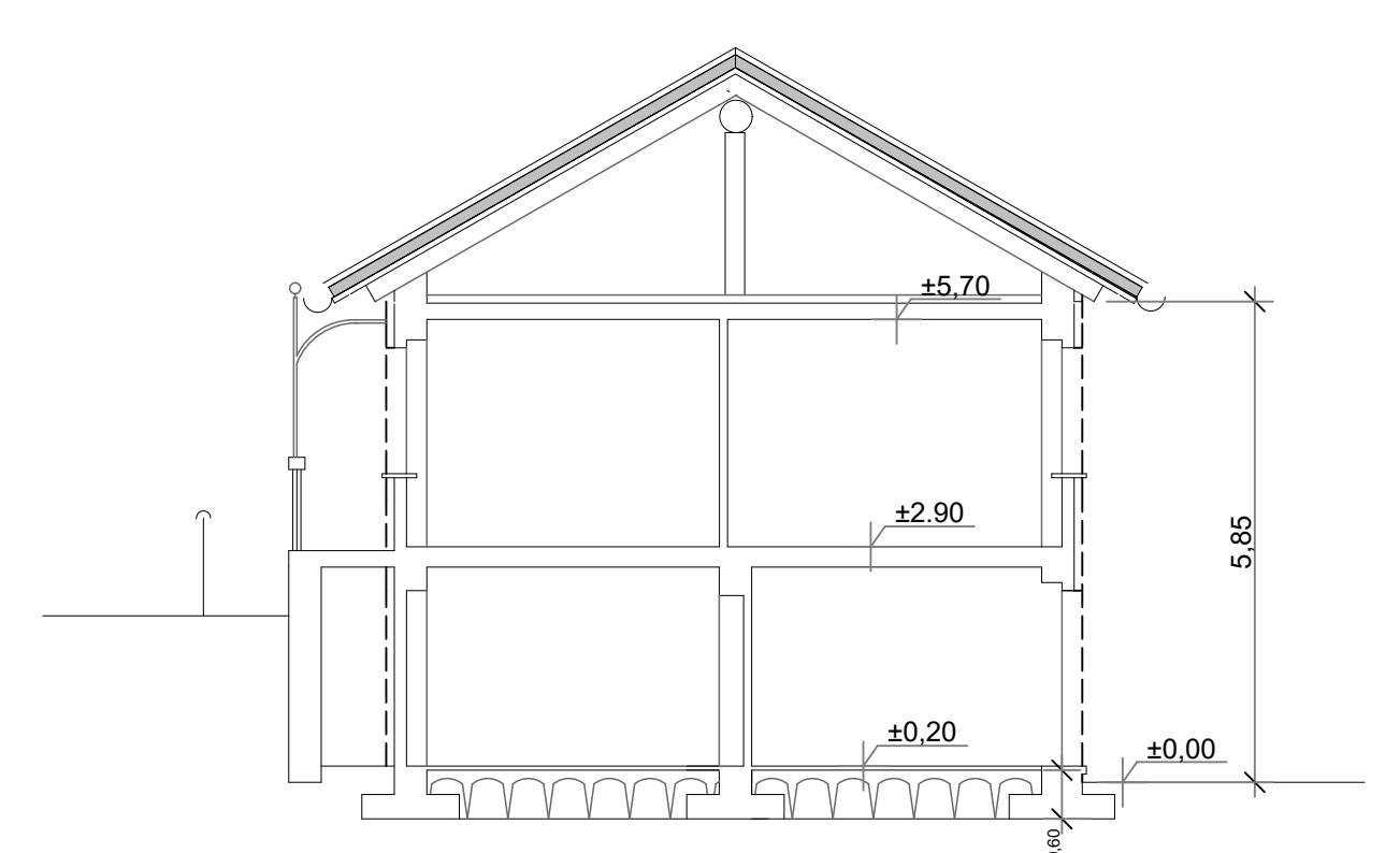
SEZIONE X - X' IN PROGETTO scala 1/100
