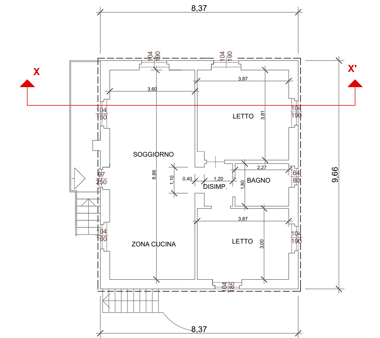
PLANIMETRIA IN PROGETTO PIANO PRIMO scala 1/100
