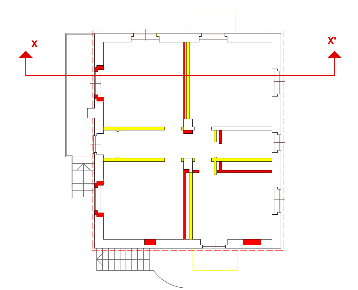
PLANIMETRIA COMPARATIVA PIANO PRIMO scala 1/100
