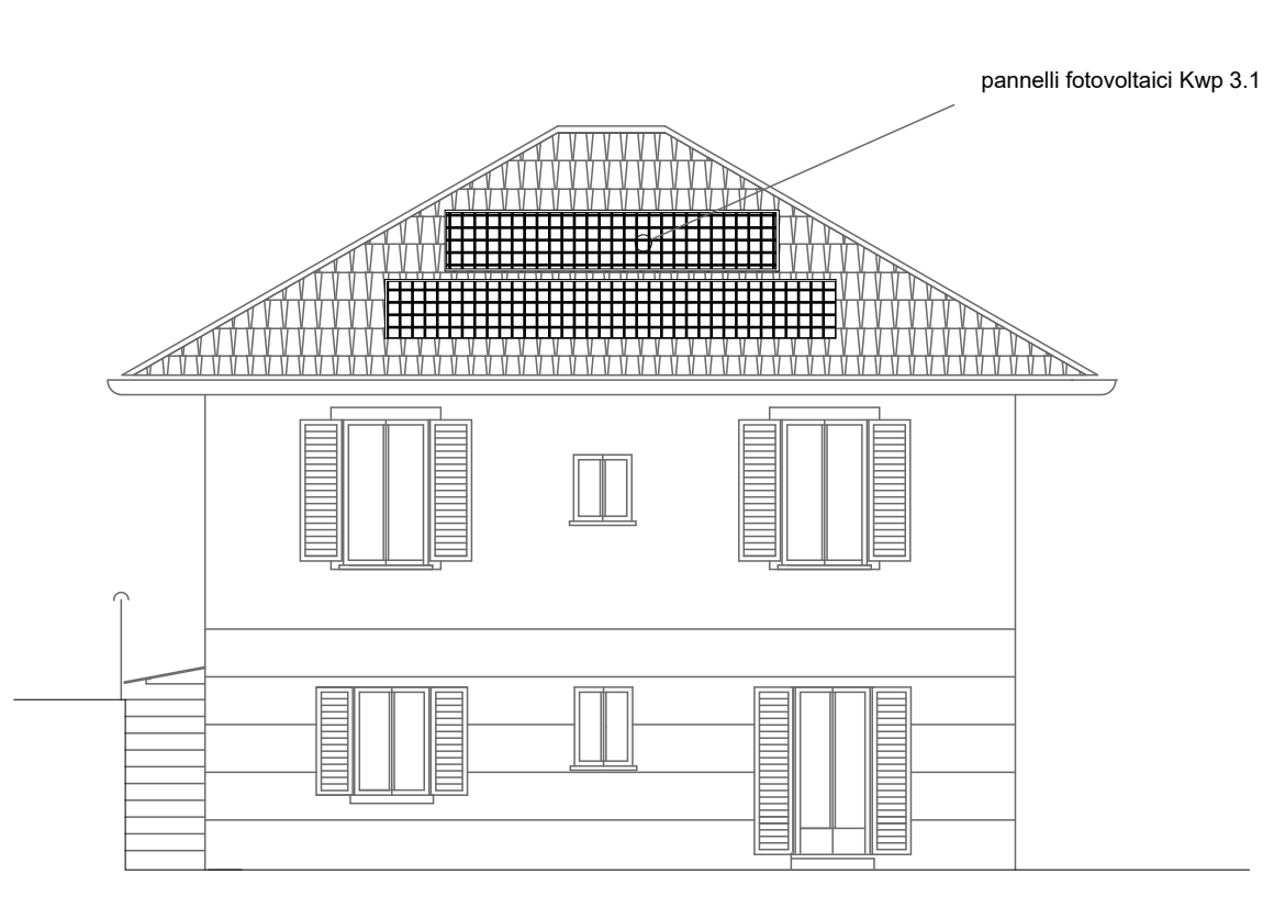
PROSPETTO EST IN PROGETTO scala 1/100
