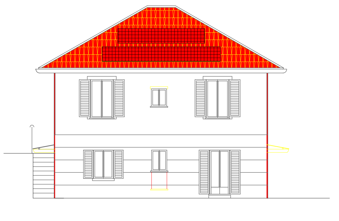
PROSPETTO EST COMPARATIVA scala 1/100
