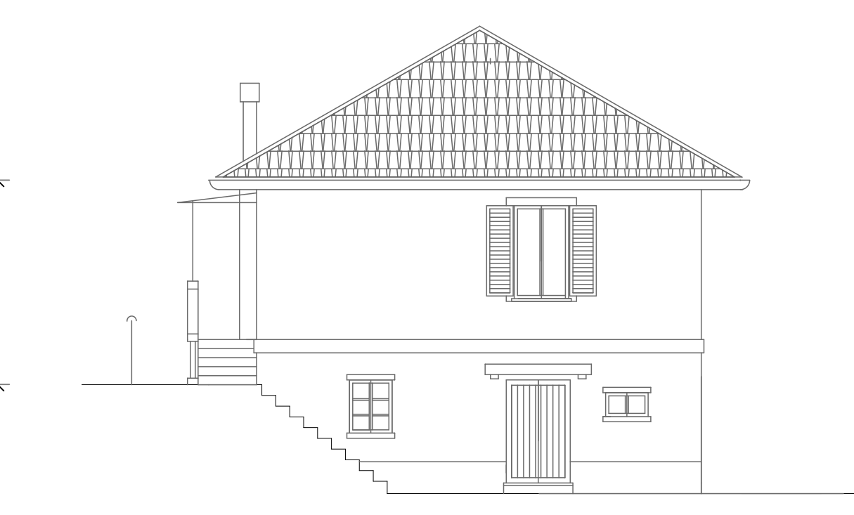
PROSPETTO SUD ESISTENTE scala 1/100
