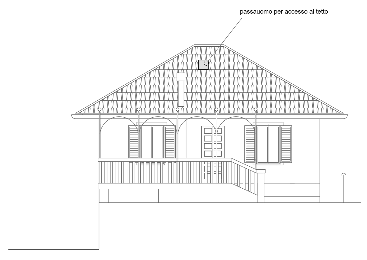
PROSPETTO OVEST IN PROGETTO scala 1/100
