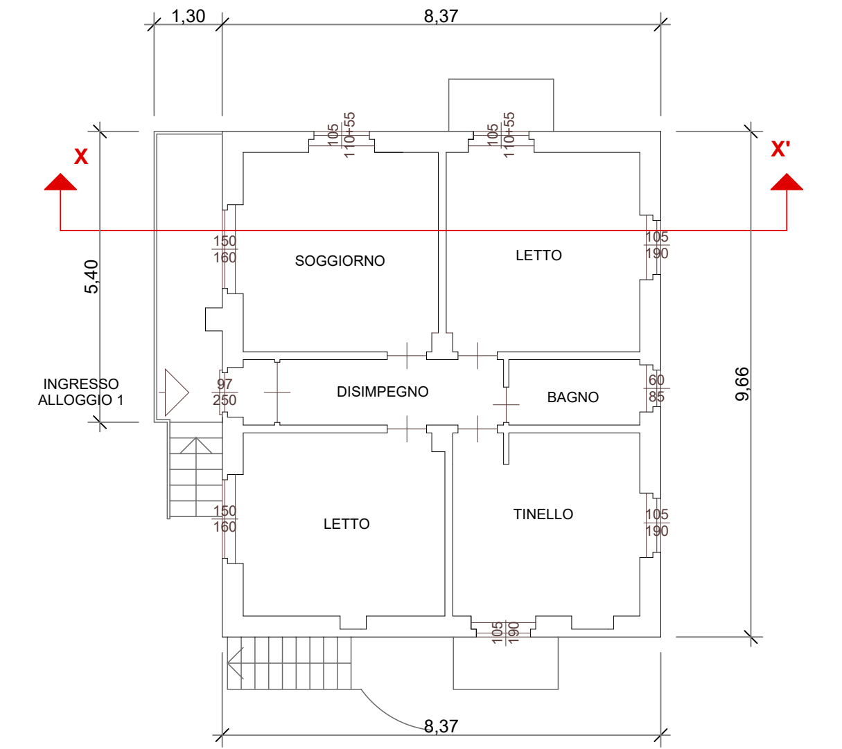
PLANIMETRIA ESISTENTE PIANO PRIMO scala 1/100
