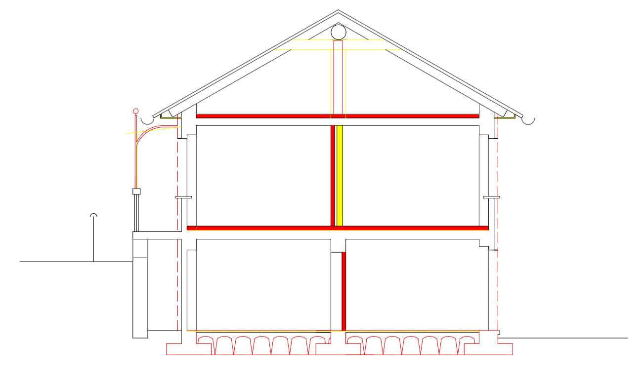
SEZIONE X - X' COMPARATIVA scala 1/100
