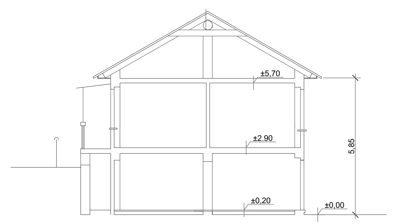
SEZIONE X - X' ESISTENTE scala 1/100
