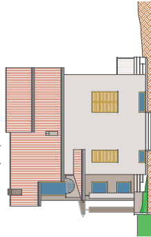
prospetto OVEST
