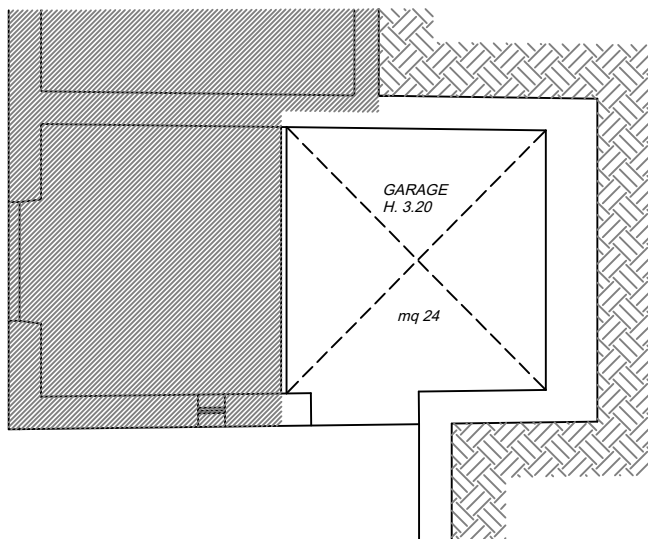
PIANTA PIANO SEMINTERRATO
