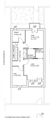
Planimetria Piano Primo sub 7
