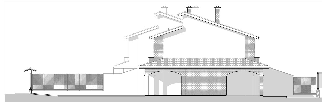
PROSPETTO SUD OVEST - EDIFICIO 2 - Scala 1:210
