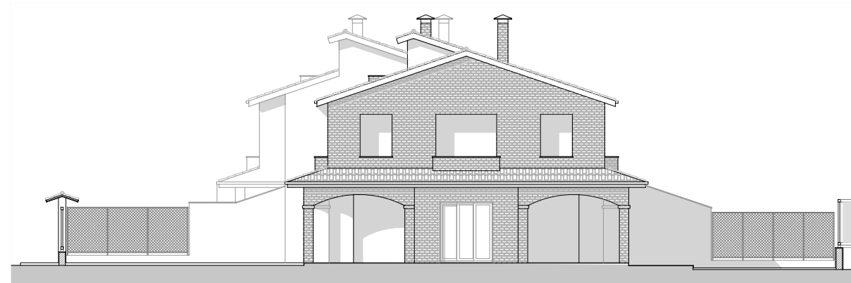
PROSPETTO SUD OVEST - EDIFICIO 1 - Scala 1:210
