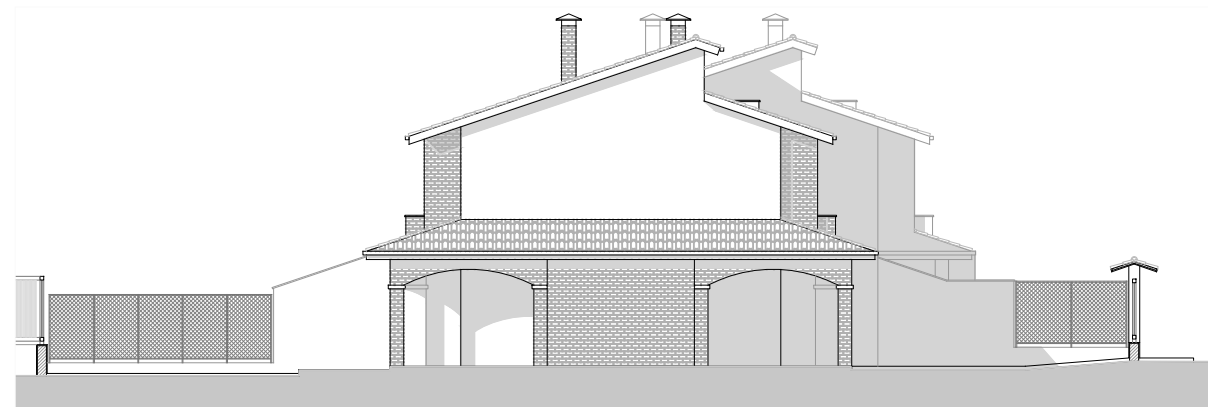
PROSPETTO NORD EST - EDIFICIO 1 - Scala 1:210
