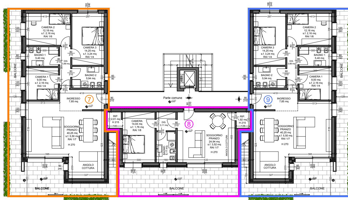
PIANTA PIANO SECONDO H 2,70 m
