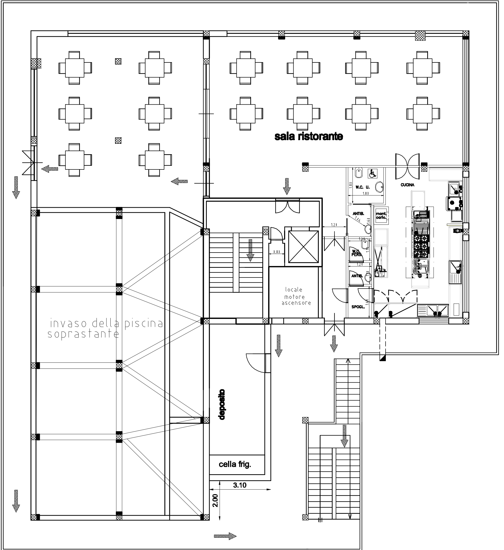
PIANTA PIANO 4°
