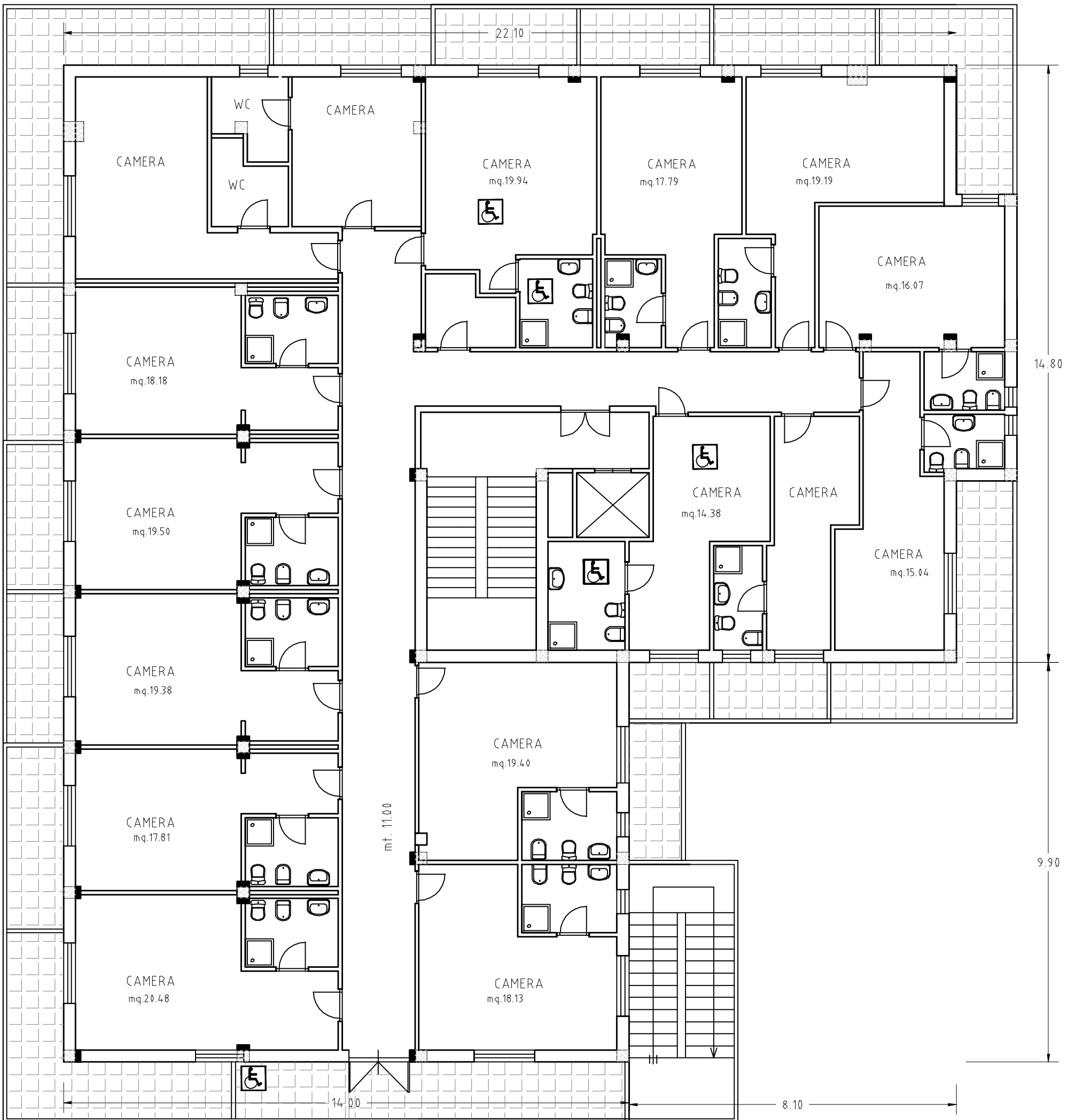
PIANTA PIANO 3°
