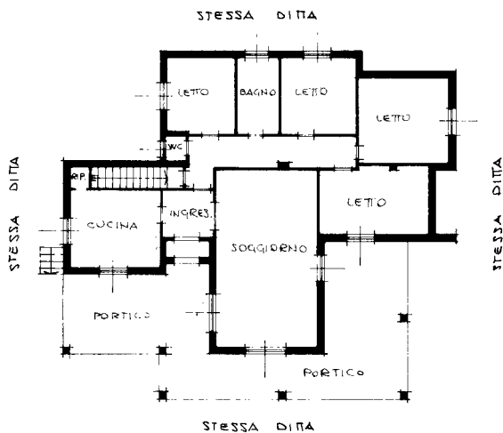
PIANO TERRA H. 300
