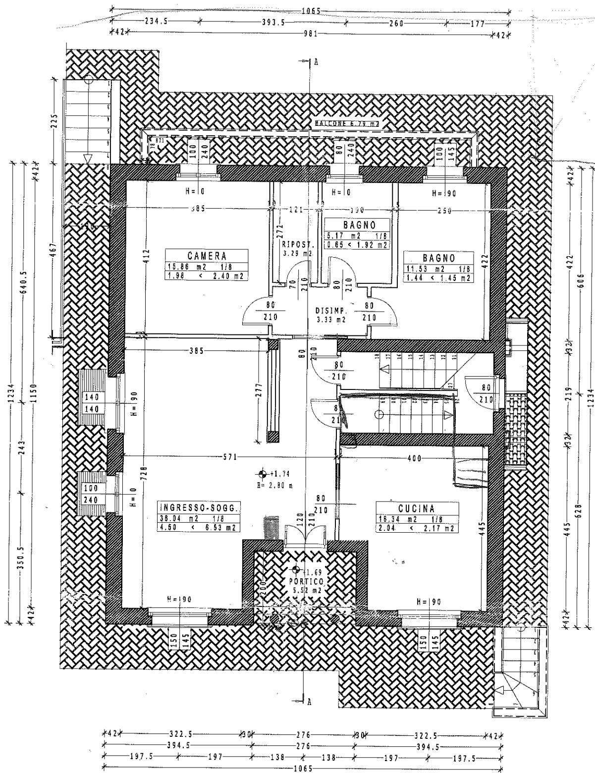
PIANTA PIANO TERRA DI VARIANTE
