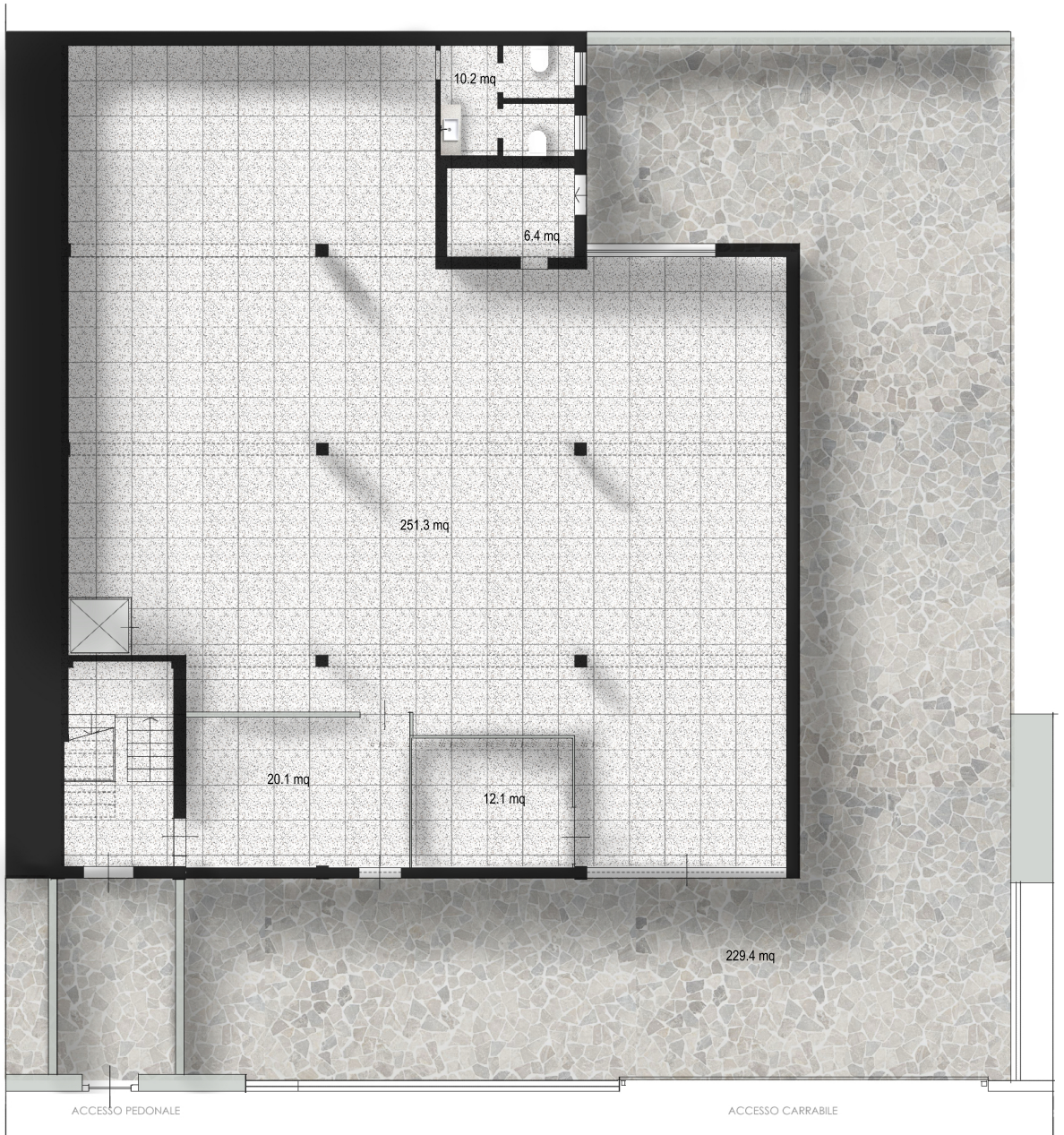
PIANTA PIANO TERRENO
