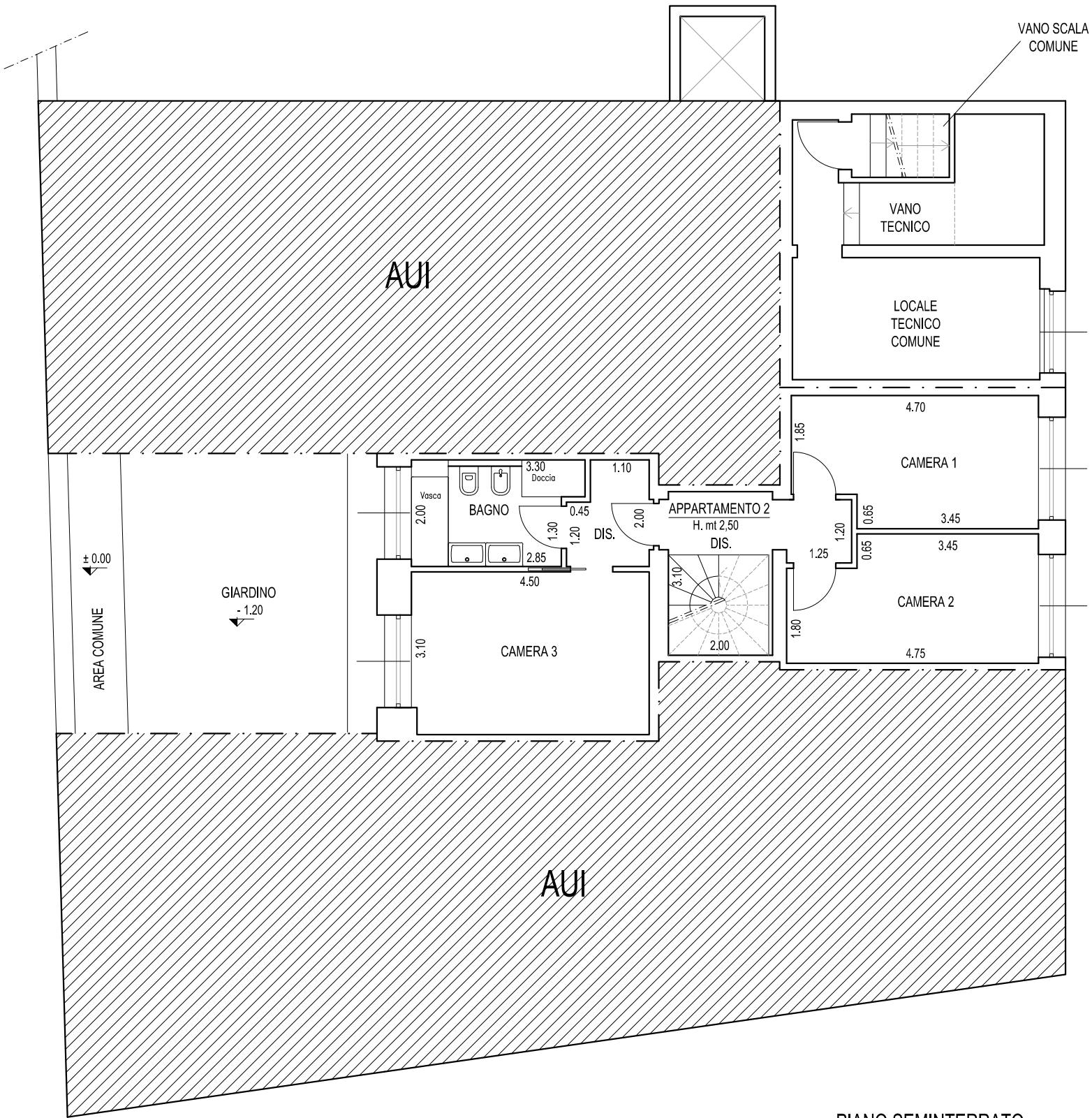
PIANO SEMINTERRATO APPARTAMENTO 2
