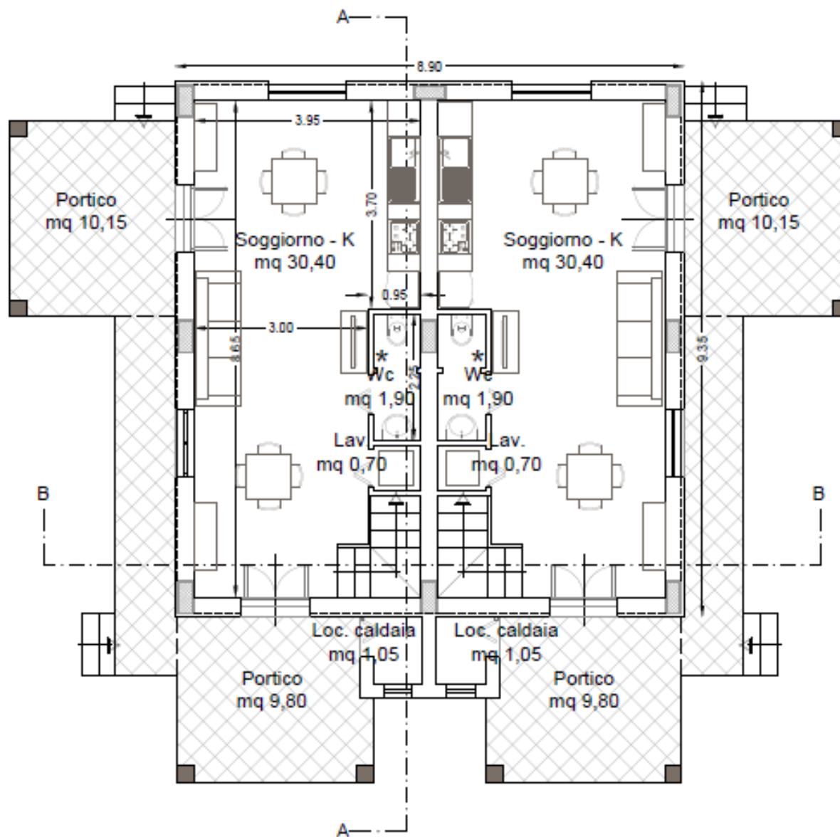
PIANTA PIANO TERRA (*) AERAZIONE FORZATA
