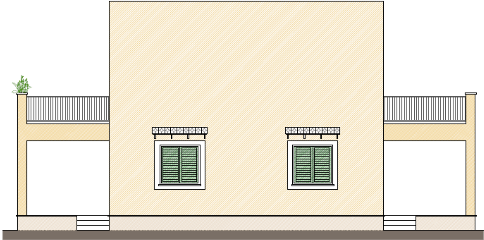
PROSPETTO POSTERIORE
